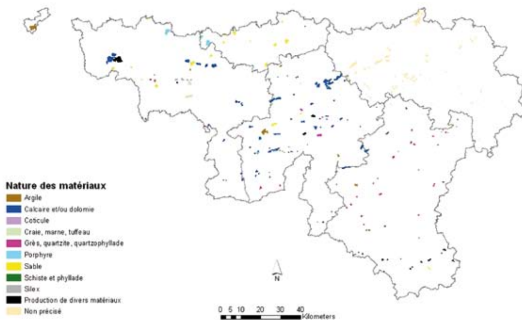
Carte des carrières en activité par type de matériau extrait (Poty 2001)
